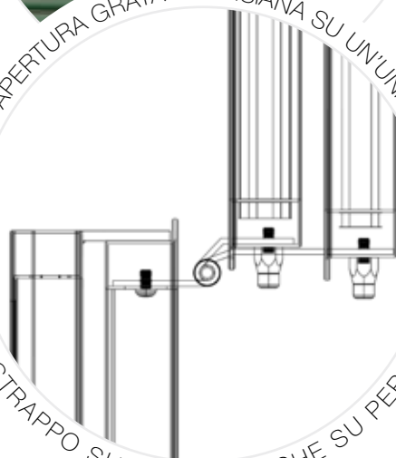
DETTAGLIO CON PERSIANA APERTA
