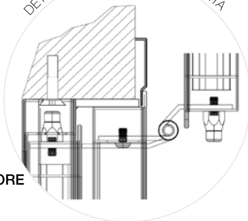
DETTAGLIO CON PERSIANA APERTA
